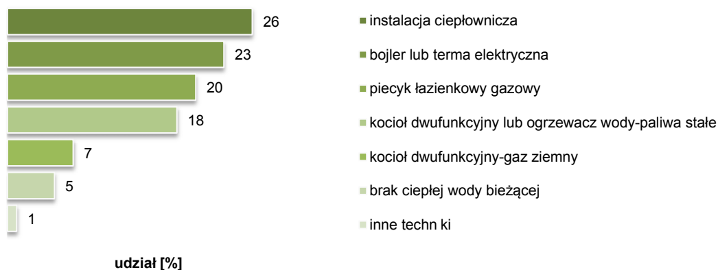
Rysunek 8. Sposoby przygotowania ciepłej wody użytkowej 14)
